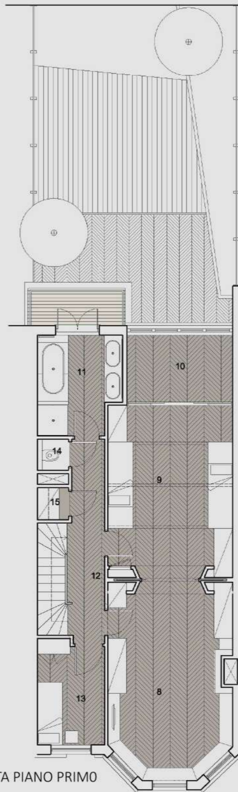
PIANTA PIANO SECONDO
